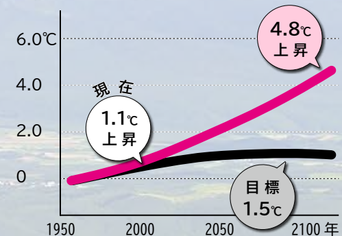
予想される世界の平均気温
