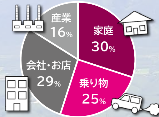
富良野市のCO 2 排出量（2019年）
