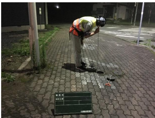
漏水調査の状況
