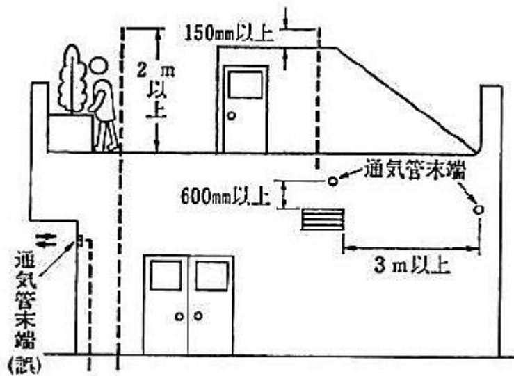
図 2-10 図 2-11 通気管の末端の開口位置 (下水道排水設備指針と解説：日本下水道協会)
