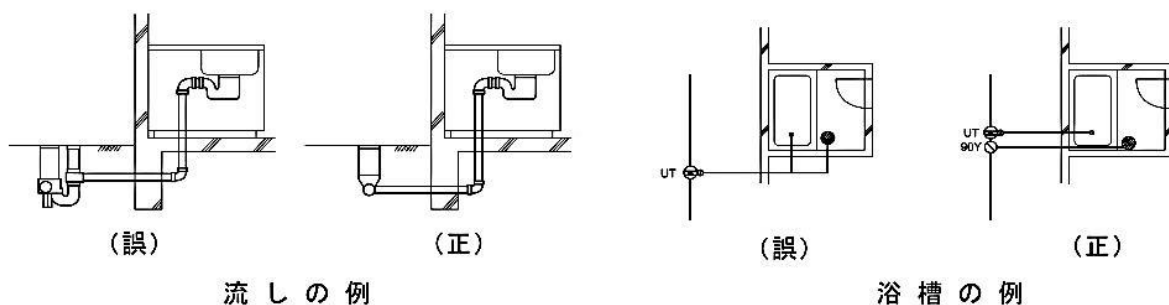
図2-19 二重トラップの事例
