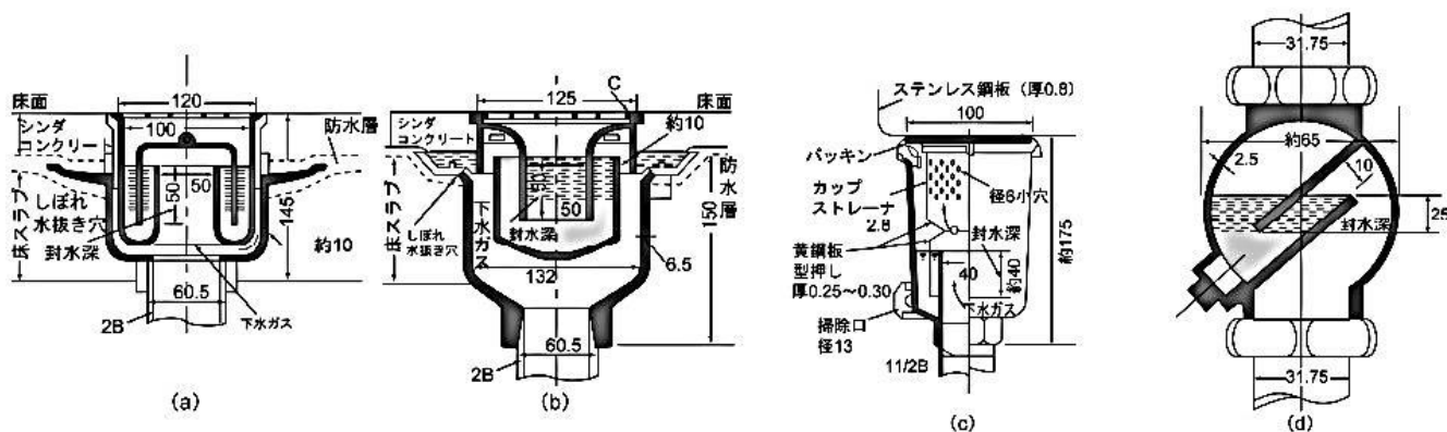
図2-17 望ましくないトラップの例 (下水道排水設備指針と解説：日本下水道協会)
