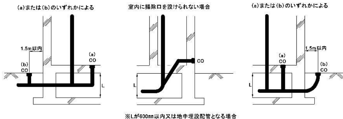
図2-7 掃除口取付け位置の例
