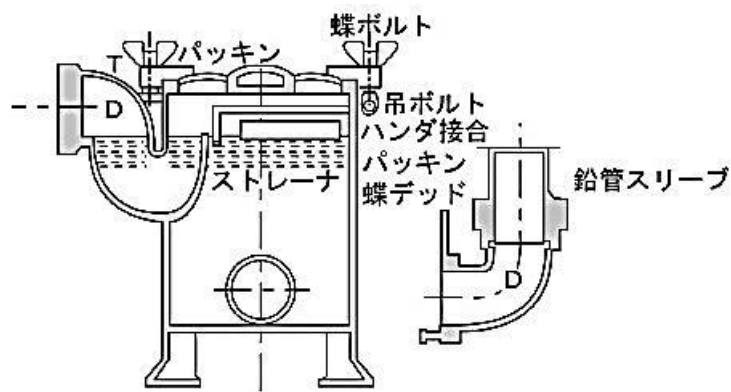
図 2-20 ドラムトラップの例 (機械設備工事監理指針：公共建築協会)
