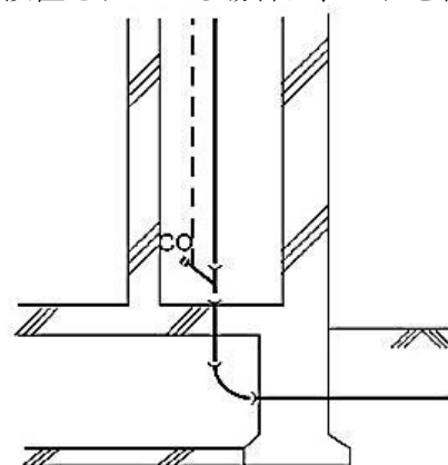
図2-8 通気管接続部の掃除口
