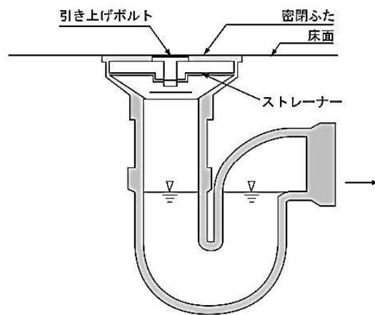
図 2-28 掃除口兼用床排水トラップ (下水道排水設備指針と解説：日本下水道協会)
