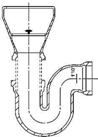
図 2-6 水受け容器 (漏斗、ホoppaの例)
