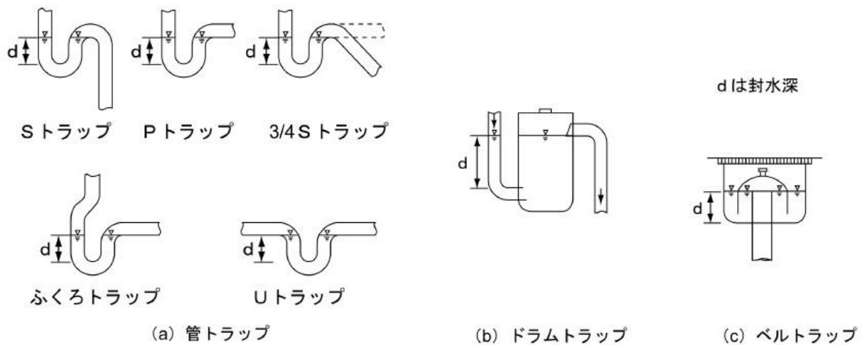
図2-14 トラップの種類 (下水道排水設備指針と解説：日本下水道協会)
