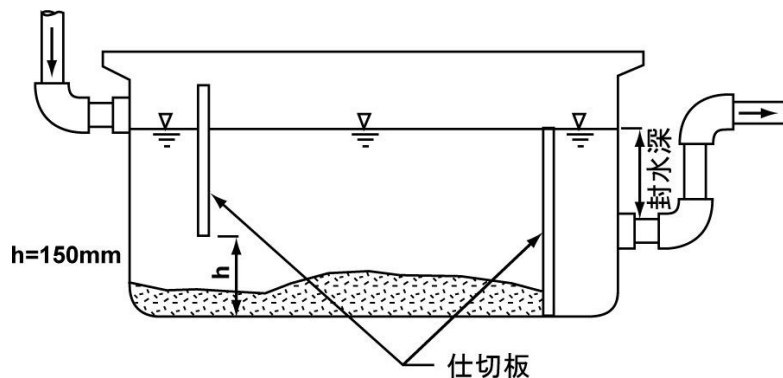
図 2-24 サンド阻集器の例 (下水道排水設備指針と解説：日本下水道協会)
