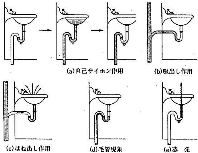
図2-15 封水破壊の原因（1）
