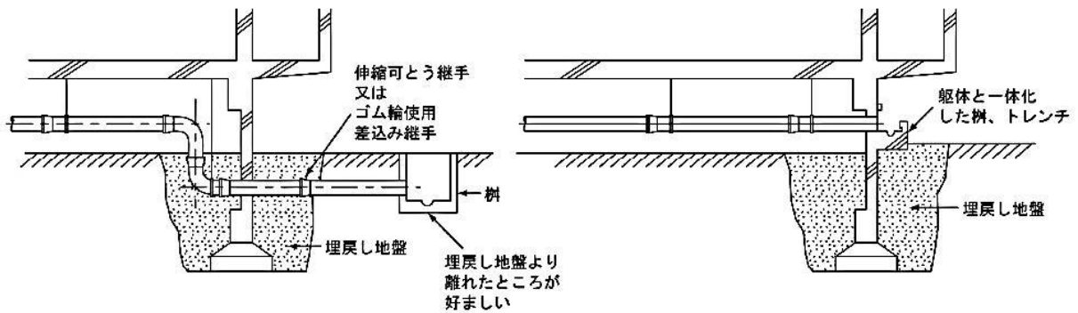
図2-5 排水管・ますの地盤沈下変位に対する対策の例 (下水道排水設備指針と解説：日本下水道協会)
