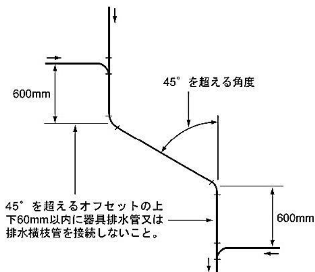
図2-2 45^\circ を超える角度をもつ オフセット部への排水横枝管の接続
