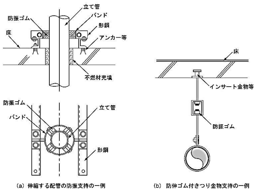
図2-4 振動を考慮した管支持方法の例 (下水道排水設備指針と解説：日本下水道協会)
