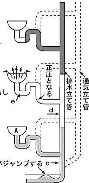
図2-16 封水破壊の原因（2）
