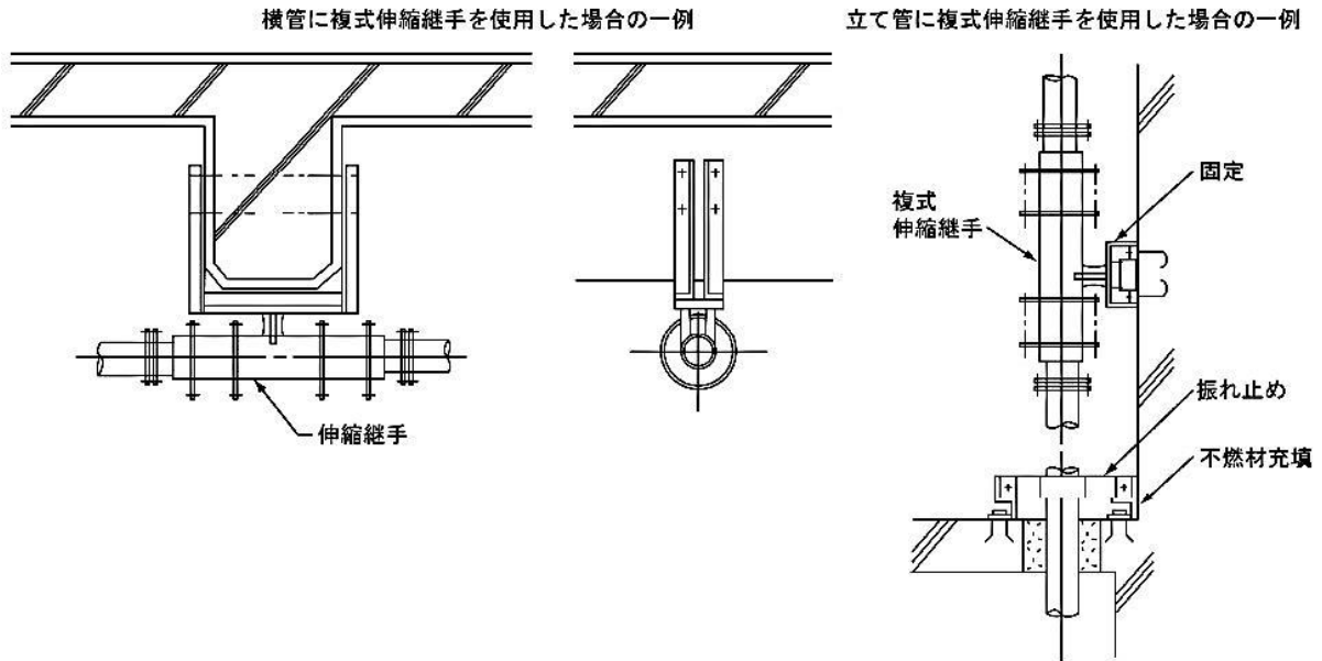
図2-3 管の損傷防止位置例 (下水道排水設備指針と解説：日本下水道協会)
