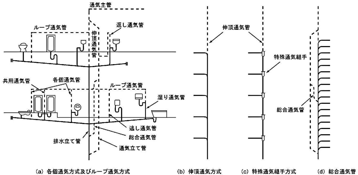
図2-9 通気管の種類と通気方式 (下水道排水設備指針と解説：日本下水道協会)
