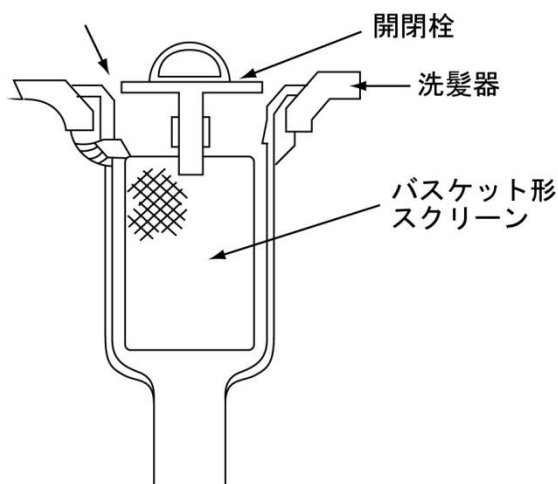
図2-25 ヘア－阻集器の一例 (下水道排水設備指針と解説：日本下水道協会)
