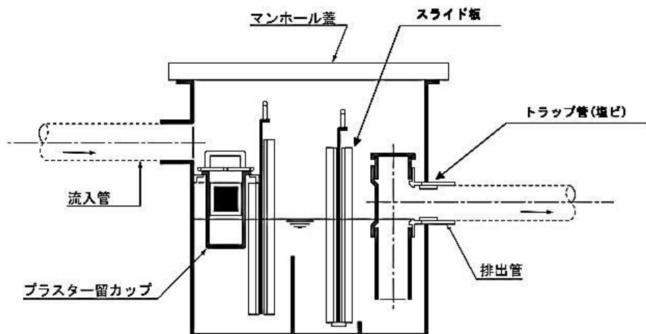
図 2-27 プラスタ（石こう）阻集器の例（下田エコテックカタログ）
