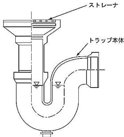
図 2-21 床排水トラップの例 (下水道排水設備指針と解説：日本下水道協会)
