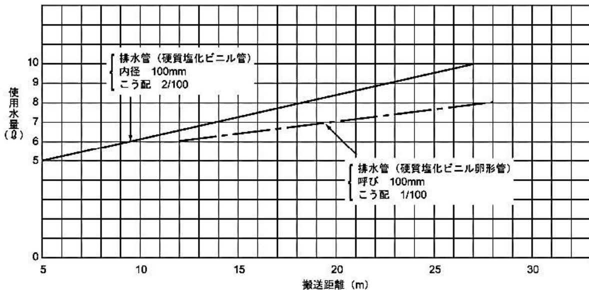
図 2-12 大便器から接続ます又は他の汚水が合流するまでの距離 (下水道排水設備指針と解説：日本下水道協会)
