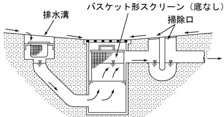
図 2-26 ランドリー用阻集器の例 (下水道排水設備指針と解説：日本下水道協会)
