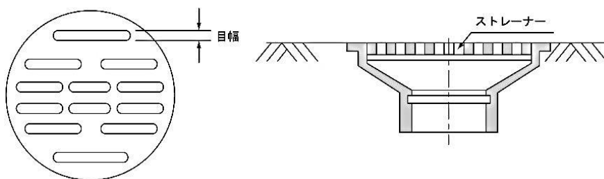
図 2-22 ストレーナの例（目皿） (下水道排水設備指針と解説：日本下水道協会)
