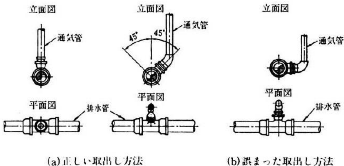
図 2-11 通気管の正しい取出し方法と誤った取出し方法 (下水道排水設備指針と解説：日本下水道協会)
