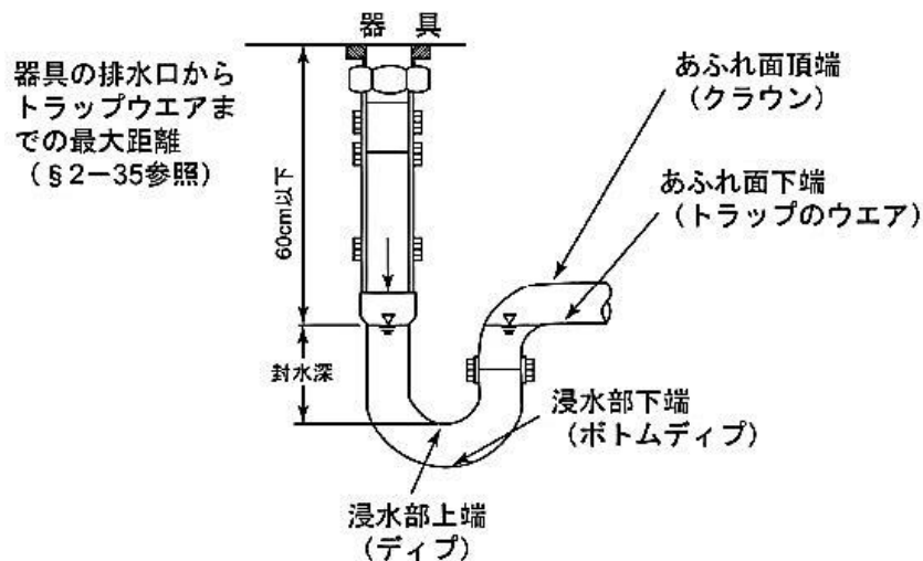
図 2-13 トラップ各部の名称 (下水道排水設備指針と解説：日本下水道協会)
