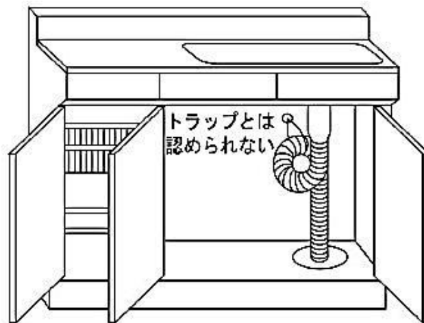
図2-18 トラップと認められない例 (東京都排水設備要綱)
