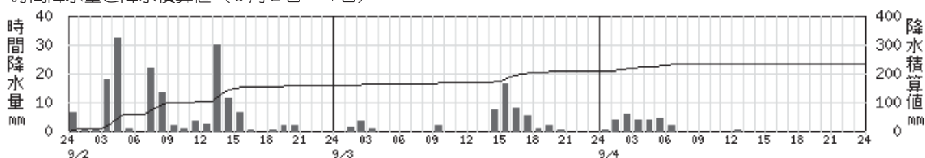
時間降水量と降水積算値（9月2日～4日）
