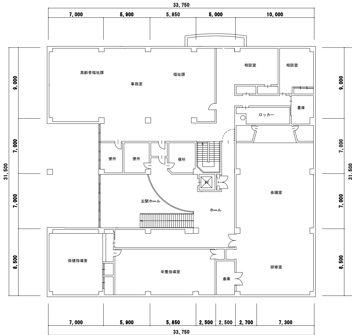
保健センター 2階平面図
