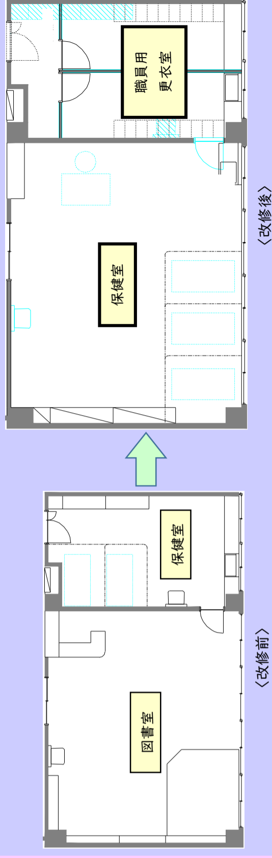
(図2) 図書室を保健室に改修, 保健室を更衣室に改修
