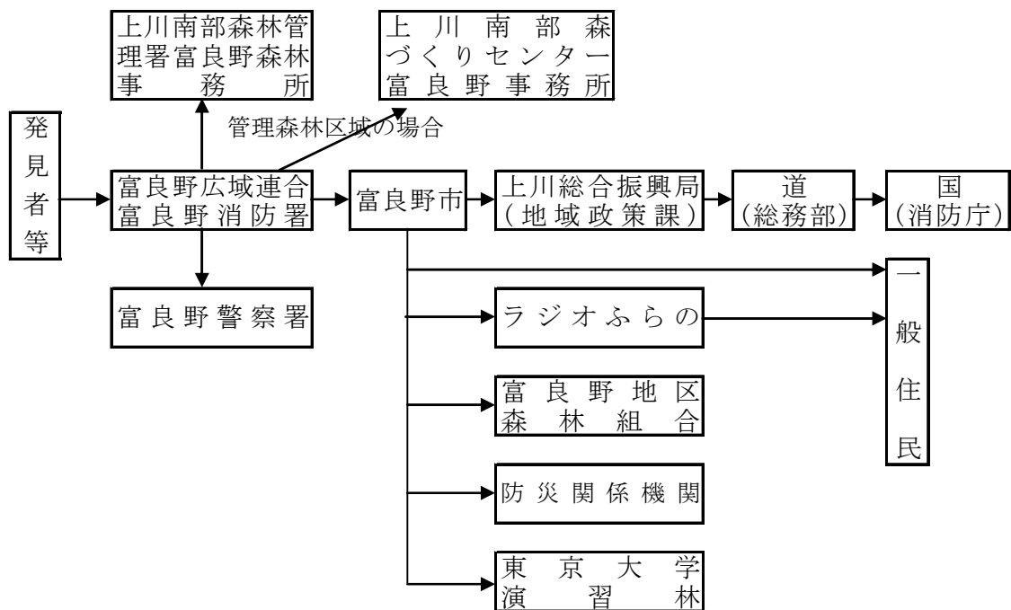
■別図7 林野火災に係る情報通信連絡系統図
