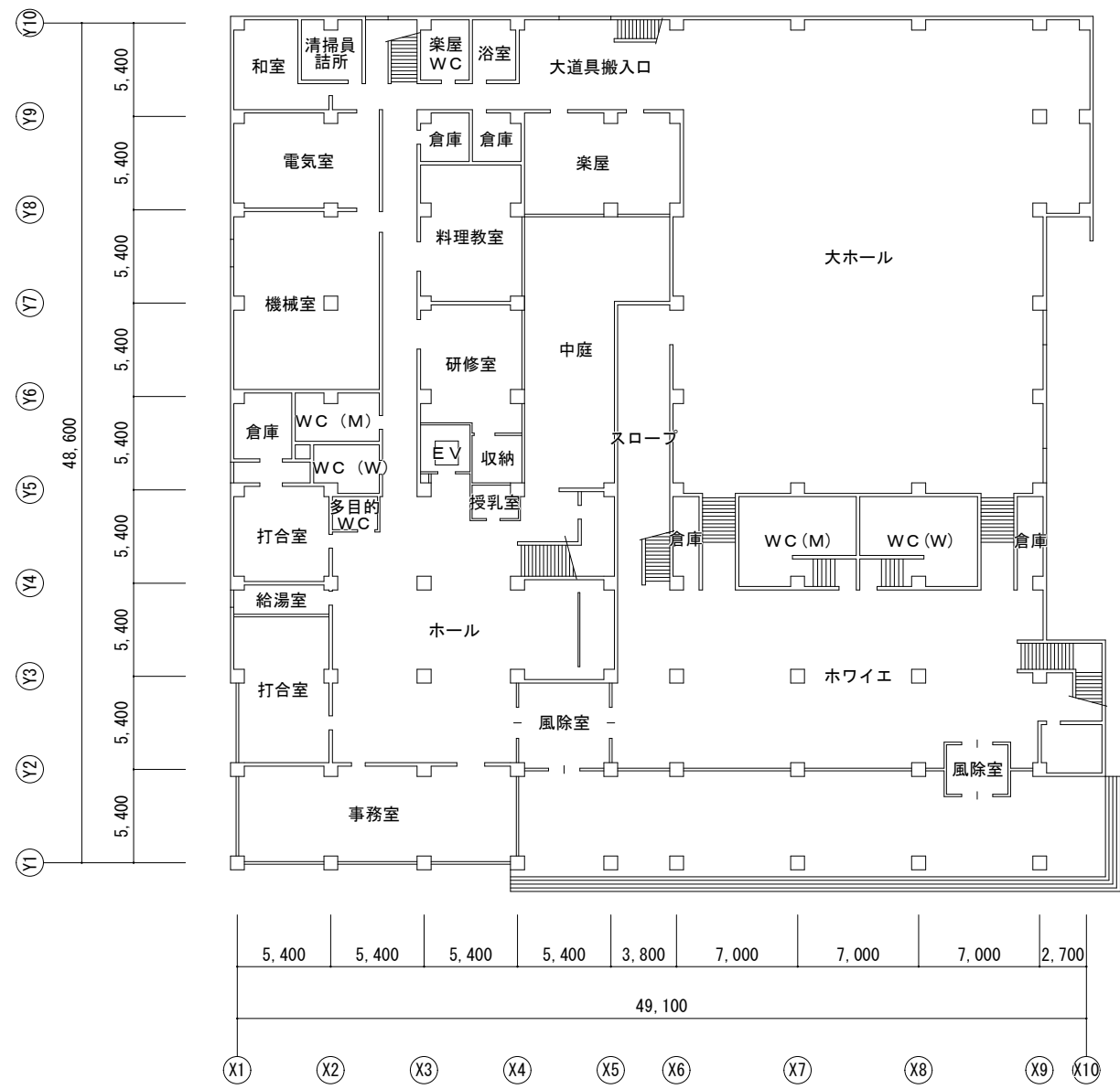
1階平面図
