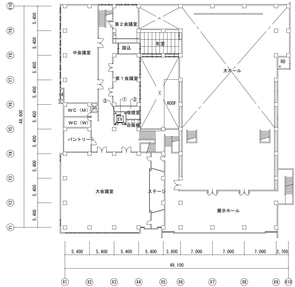
2階平面図
