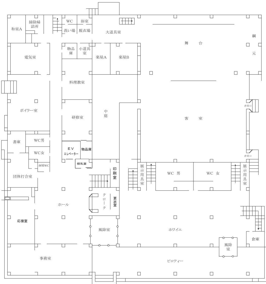
1F 平面図
